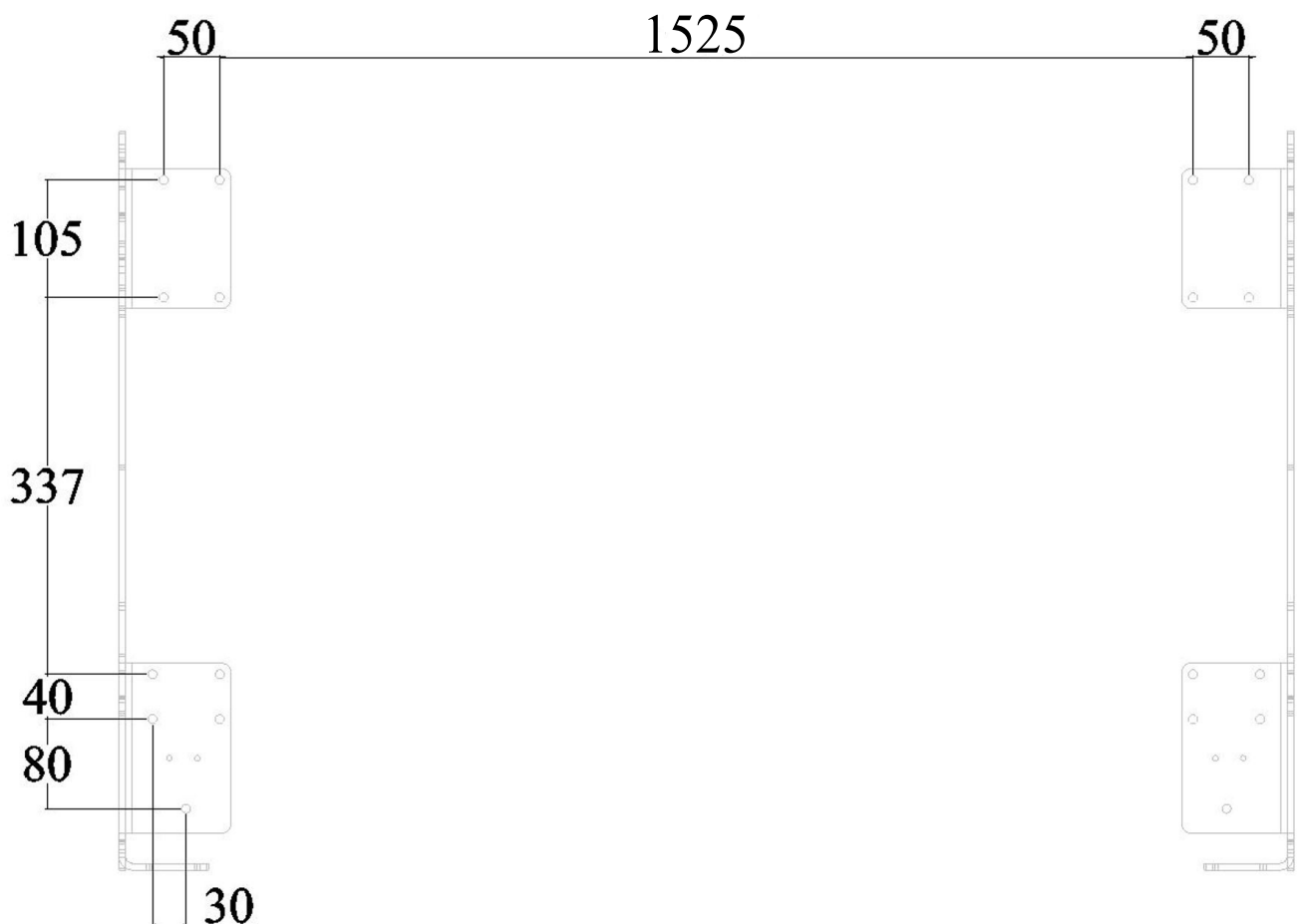
Bohrbild
